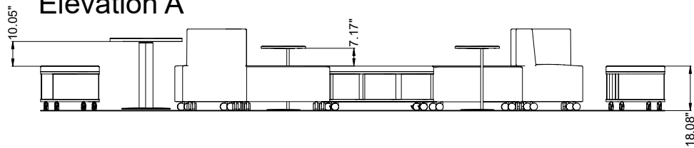
Elevation A
